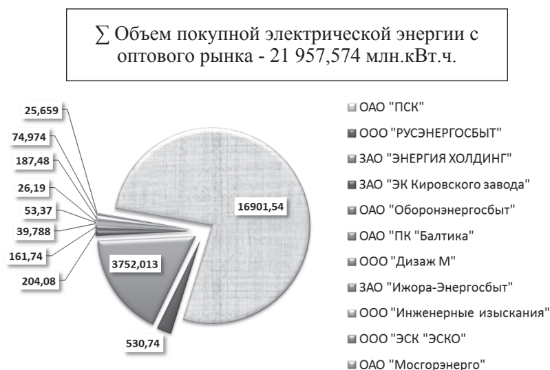
Рис. 1. Соотношение объема покупной электрической энергии с оптового рынка в Санкт-Петербурге в 2013 году.
