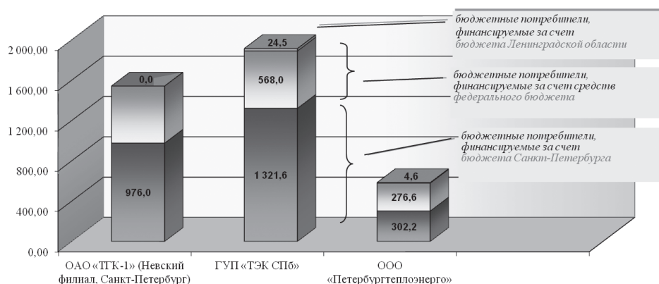
Рис. 10. Структура полезного отпуска тепловой энергии бюджетным потребителям, финансируемым за счет средств бюджетов различных уровней.
